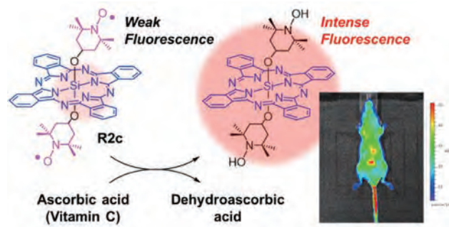
■フタロシアニンR2cを用いたマウス中におけるビタミンCの蛍光イメージング Fluorescent imaging of Vitamin C in a mouse using the phthalocyanine R2c
